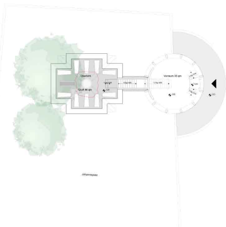
Untergeschoss M 1:100
