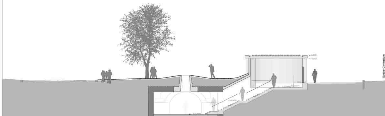
Schnitt M 1:100
